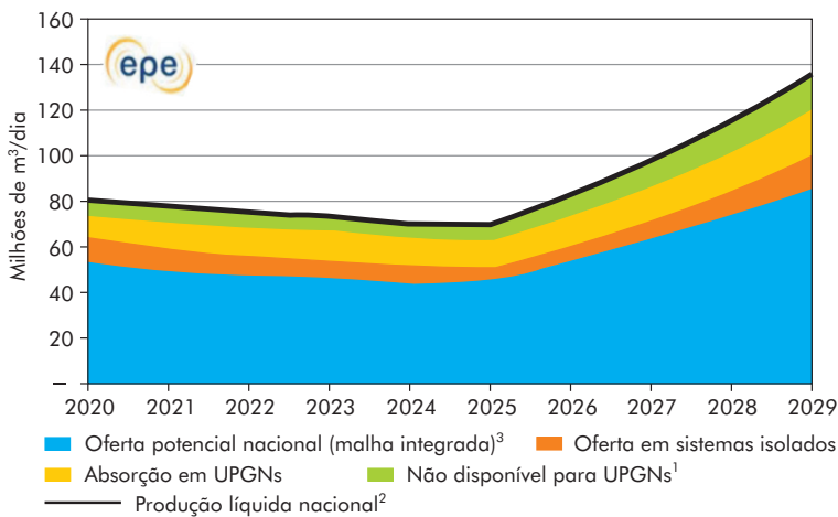
Figura 11 Perspectiva de oferta potencial nacional de gás natural (milhões de m 3 /dia)
