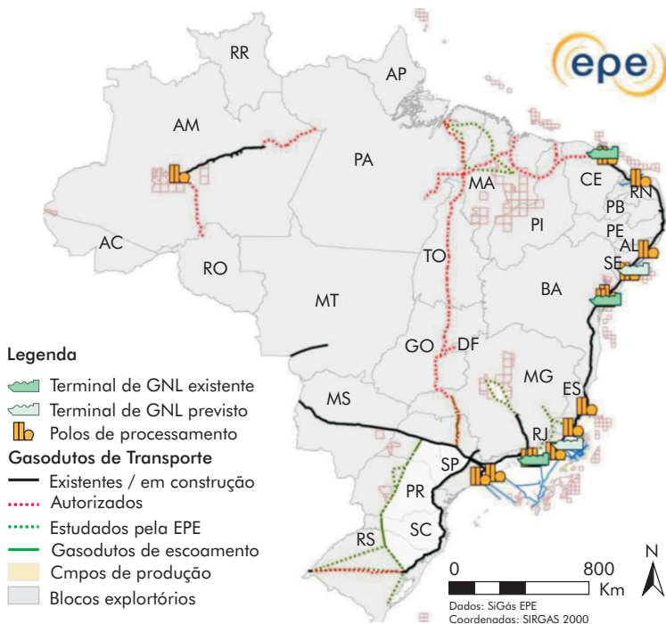
Figura 2 Infraestrutura brasileira de gás natural
