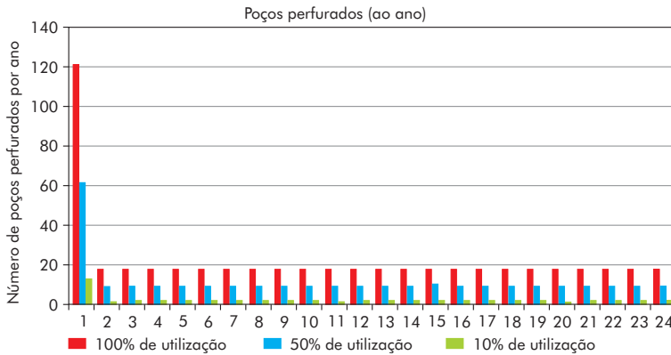
Figura 18 Número de poços perfurados ano a ano para manter o fornecimento de gás
